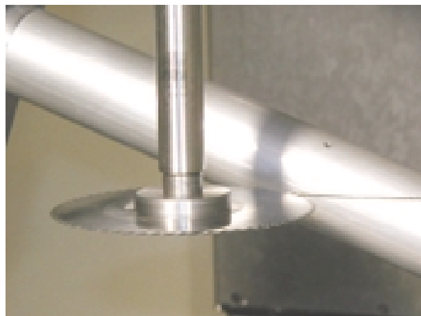
Fresatura Milling
